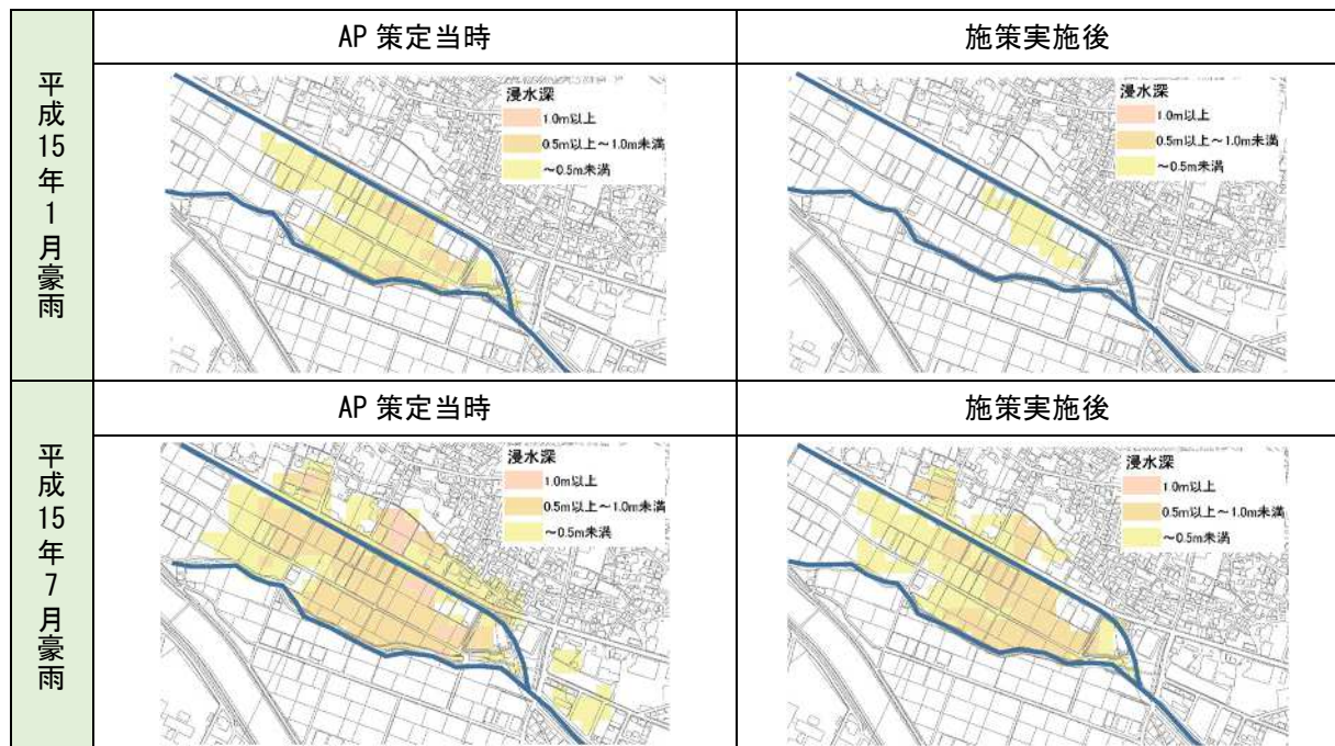
図 5.6 小潤井川・伝法沢川流域における施策効果
